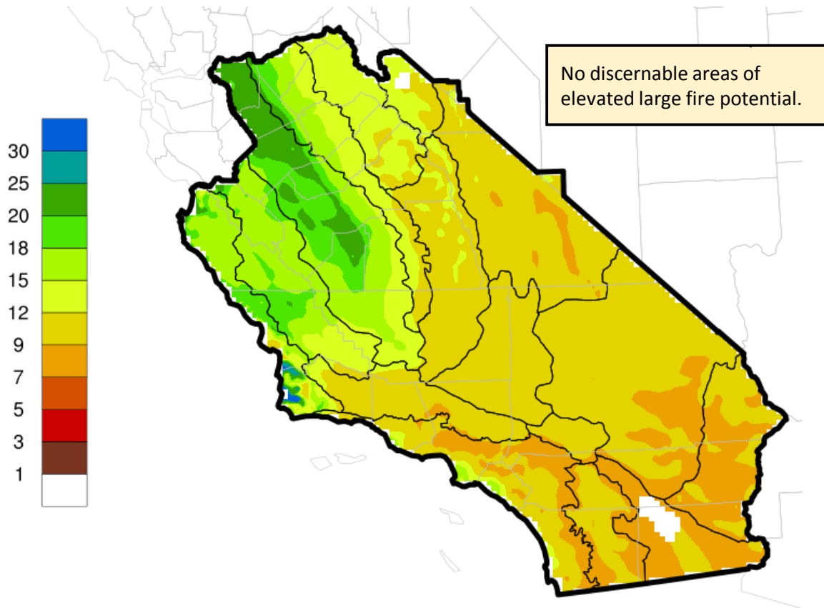
1300 LST FM10 Hour (%)
