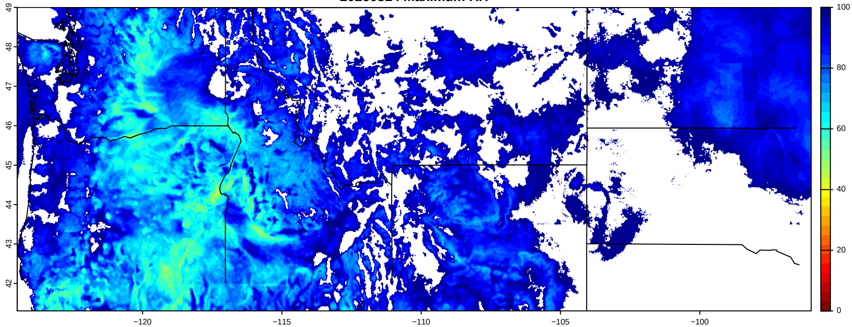
20260814 Maximum RH
